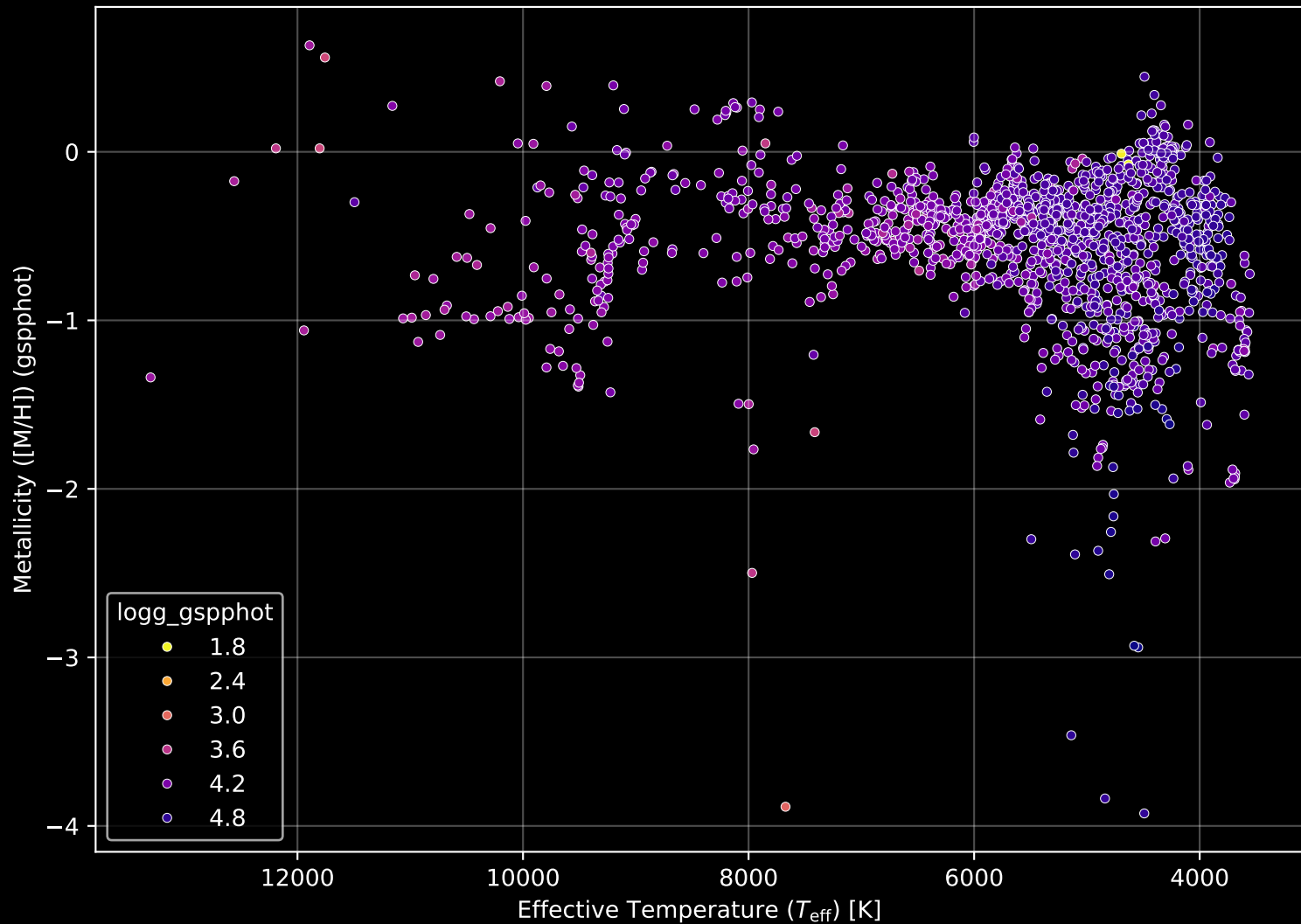
Gaia Cluster: [NGC_2168] Stellar Population Parameters (n= 1503)
