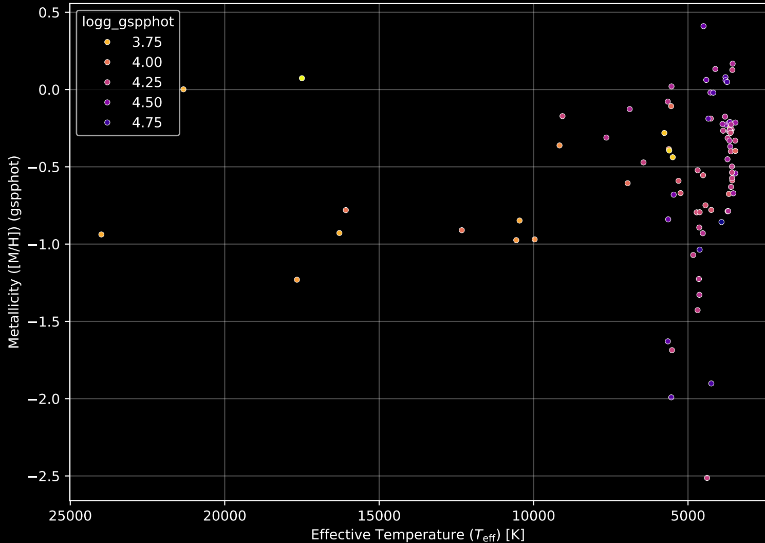
Gaia Cluster: [NGC_2169] Stellar Population Parameters (n= 91)
