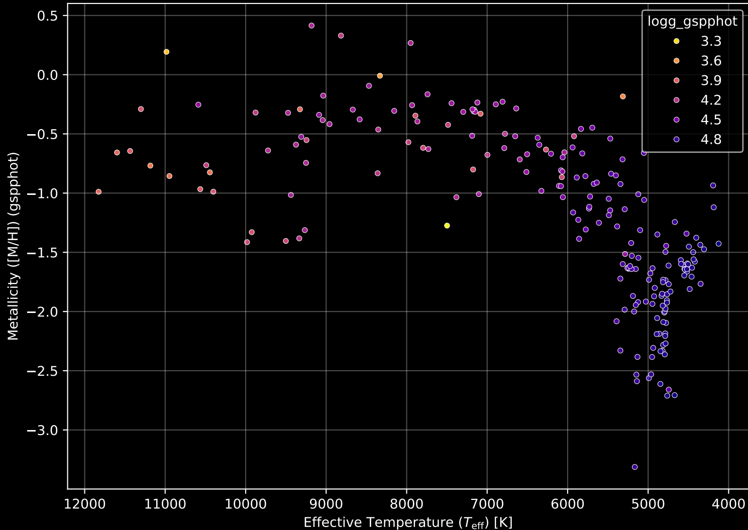
Gaia Cluster: [NGC_2186] Stellar Population Parameters (n= 210)
