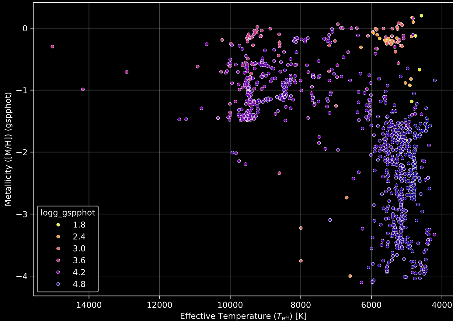
Gaia Cluster: [NGC_2194] Stellar Population Parameters (n= 1017)
