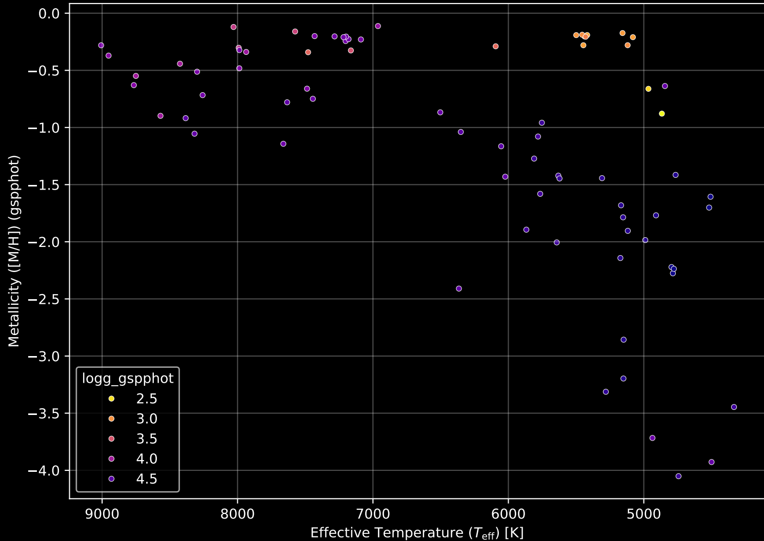
Gaia Cluster: [NGC_2225] Stellar Population Parameters (n= 76)
