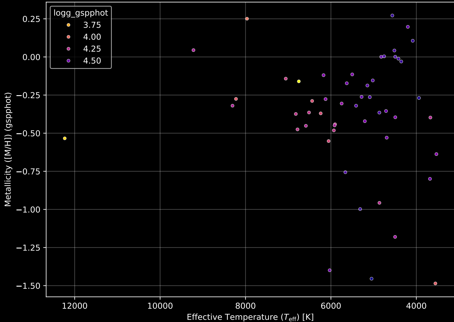
Gaia Cluster: [NGC_225] Stellar Population Parameters (n= 52)
