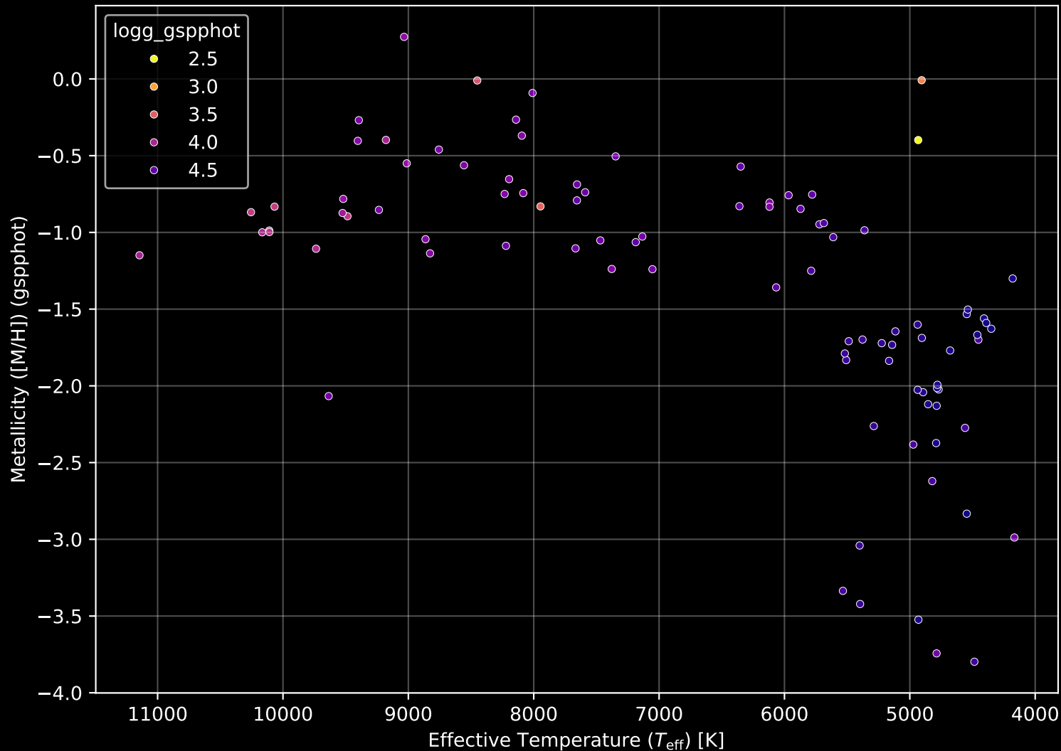
Gaia Cluster: [NGC_2269] Stellar Population Parameters (n= 94)
