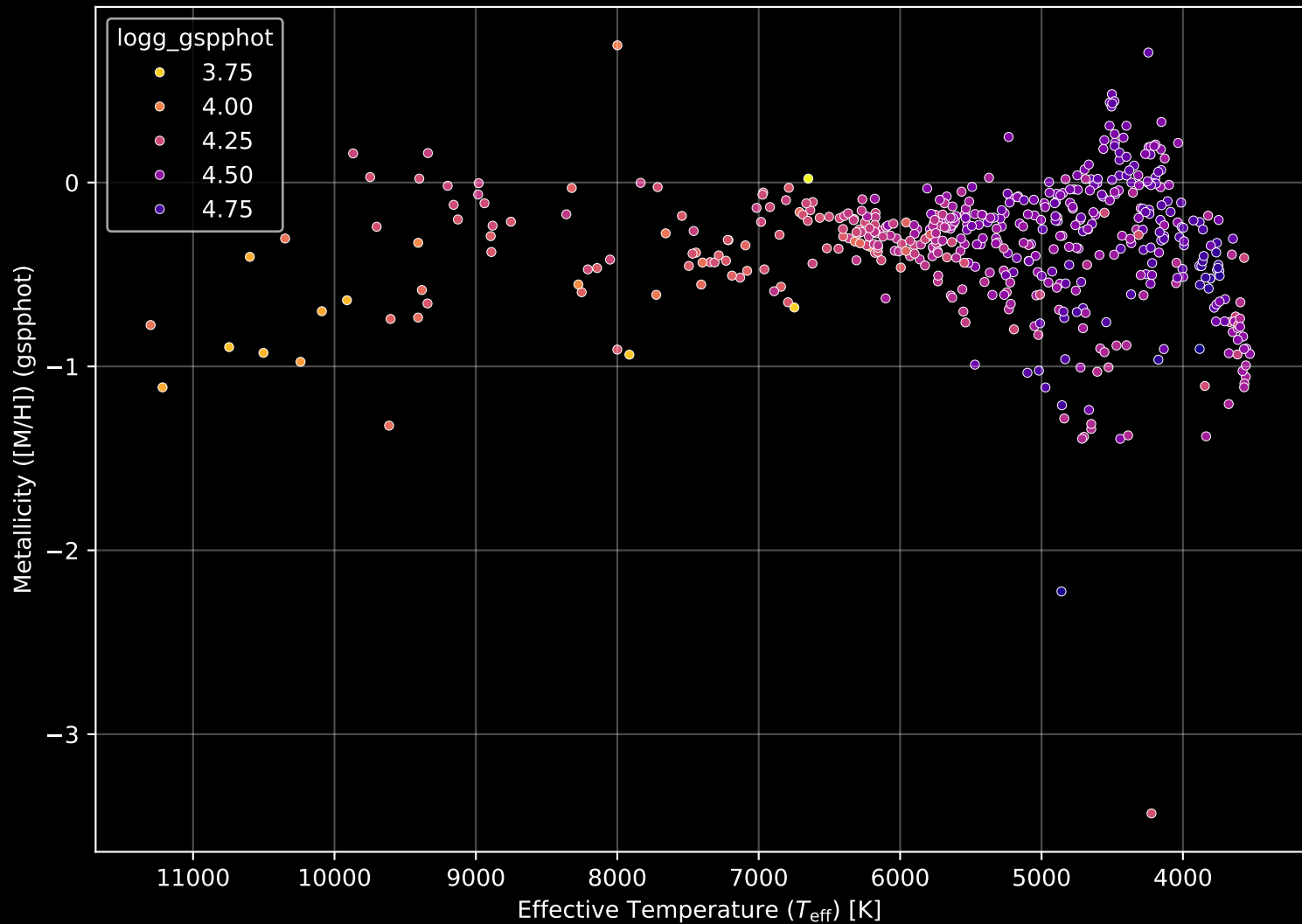
Gaia Cluster: [NGC_2301] Stellar Population Parameters (n= 516)
