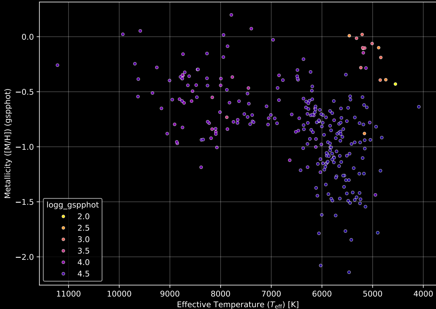
Gaia Cluster: [NGC_2304] Stellar Population Parameters (n= 260)
