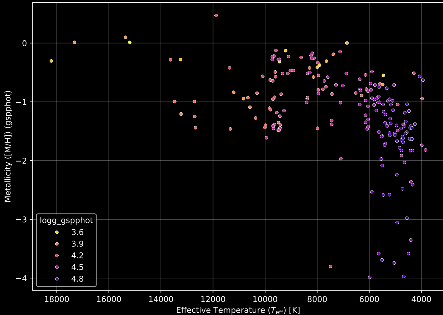
Gaia Cluster: [NGC_2311] Stellar Population Parameters (n= 204)
