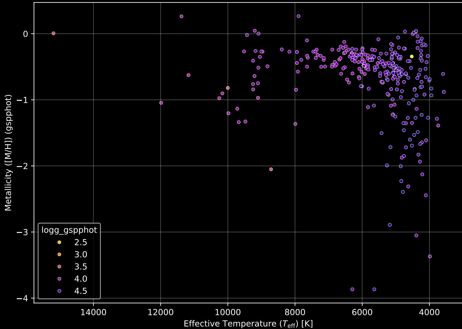
Gaia Cluster: [NGC_2353] Stellar Population Parameters (n= 289)
