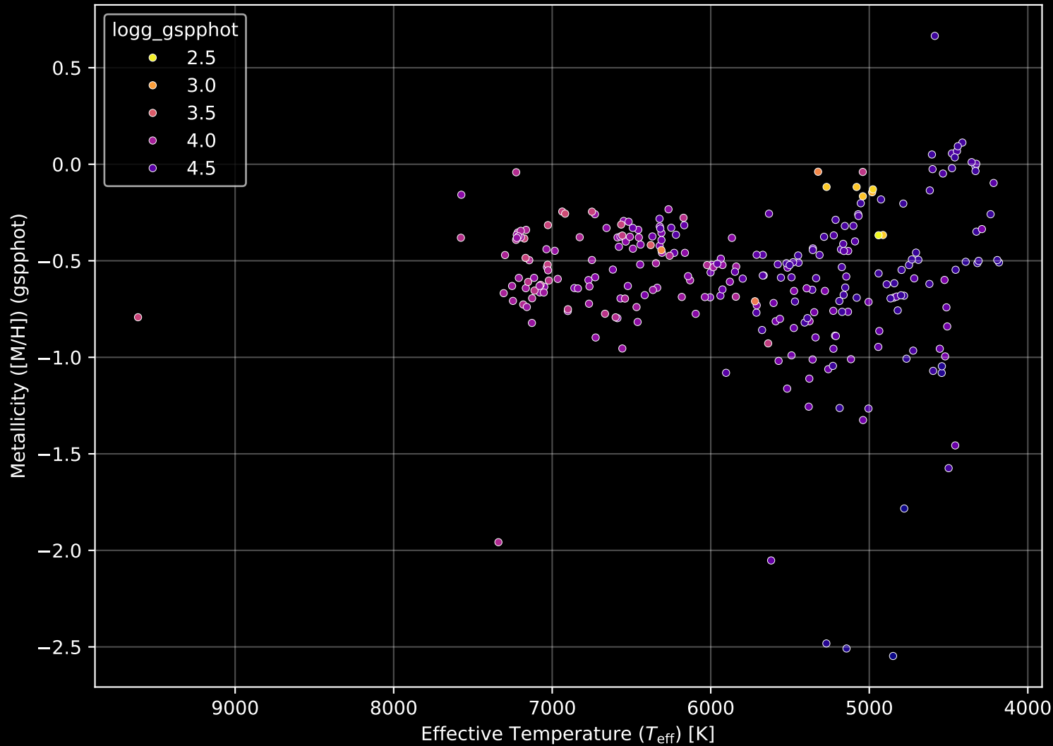
Gaia Cluster: [NGC_2354] Stellar Population Parameters (n= 273)
