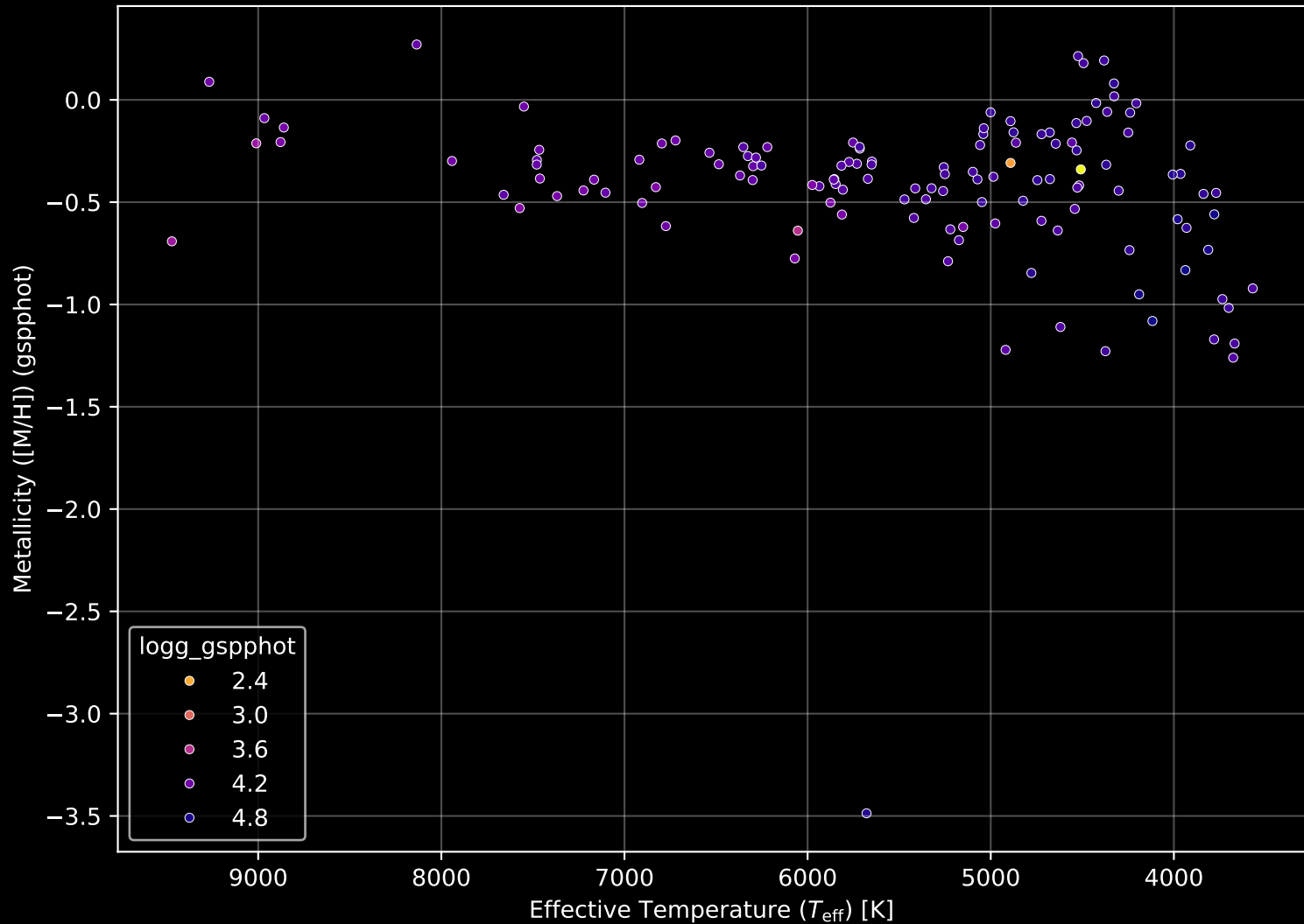
Gaia Cluster: [NGC_2358] Stellar Population Parameters (n= 131)
