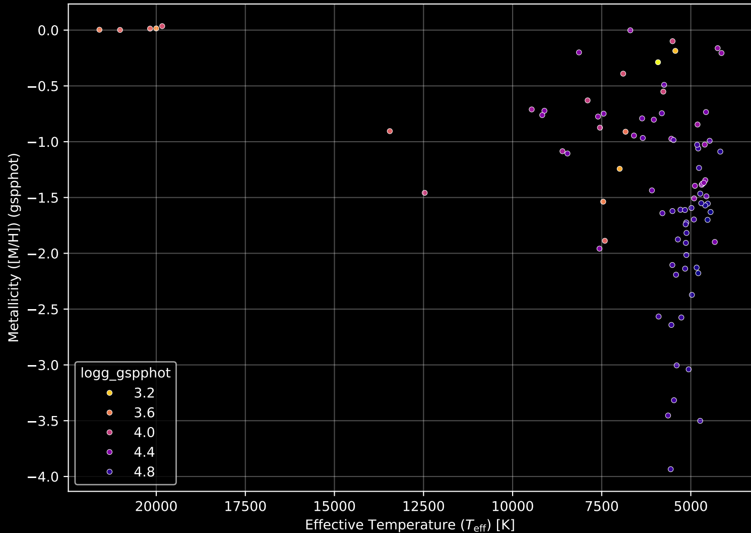
Gaia Cluster: [NGC_2367] Stellar Population Parameters (n= 89)
