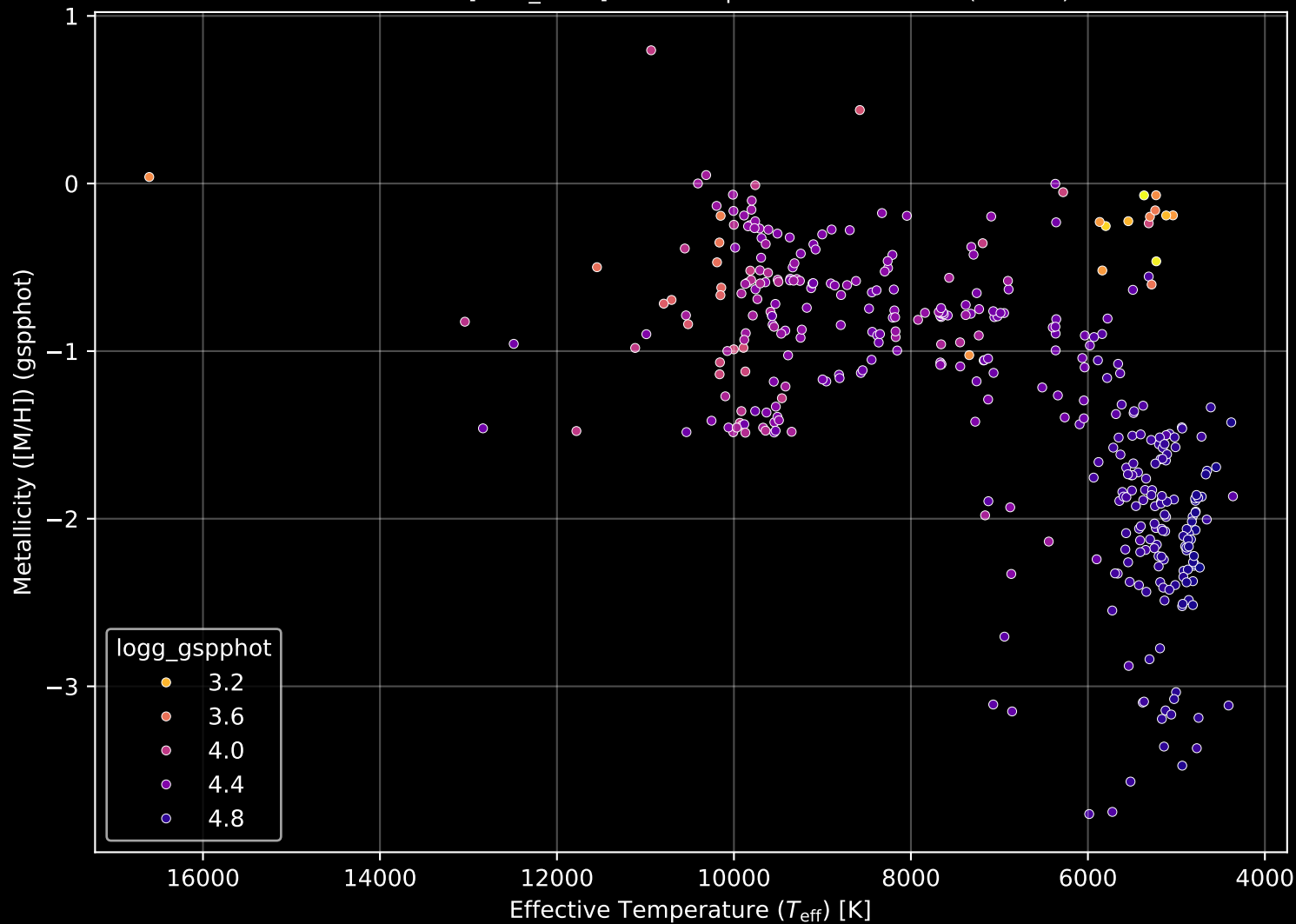
Gaia Cluster: [NGC_2383] Stellar Population Parameters (n= 387)
