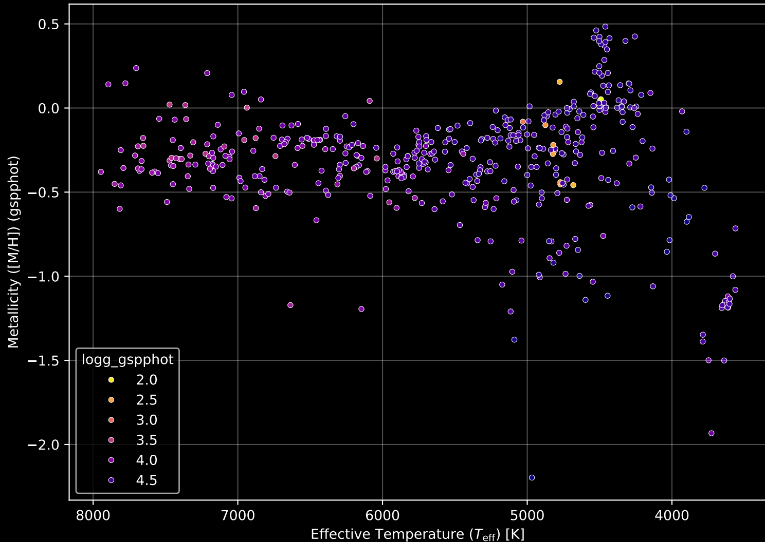
Gaia Cluster: [NGC_2423] Stellar Population Parameters (n= 462)
