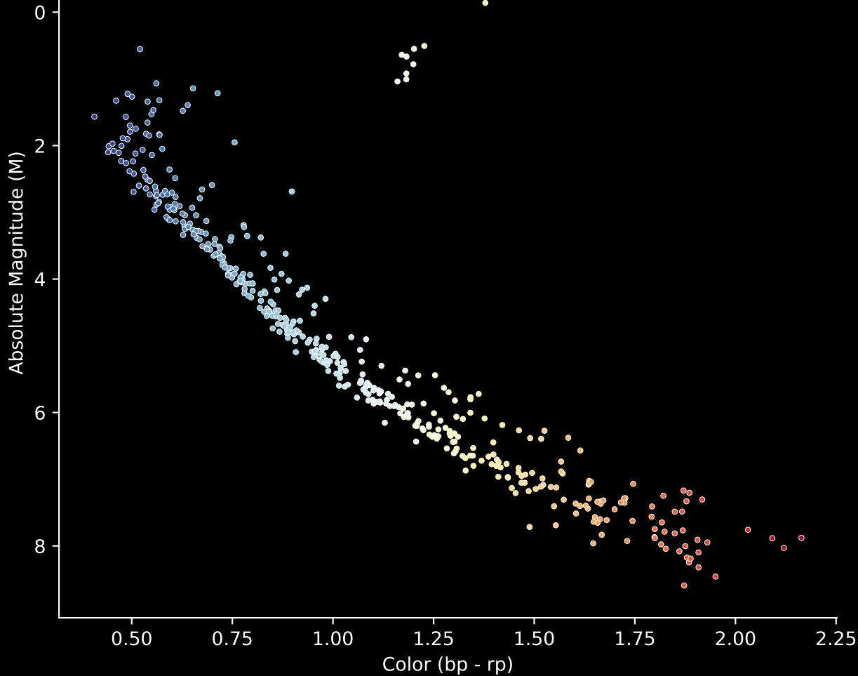
Gaia Cluster: [NGC 2423] Stars (n= 462) Hertzsprung-Russel Diagram
