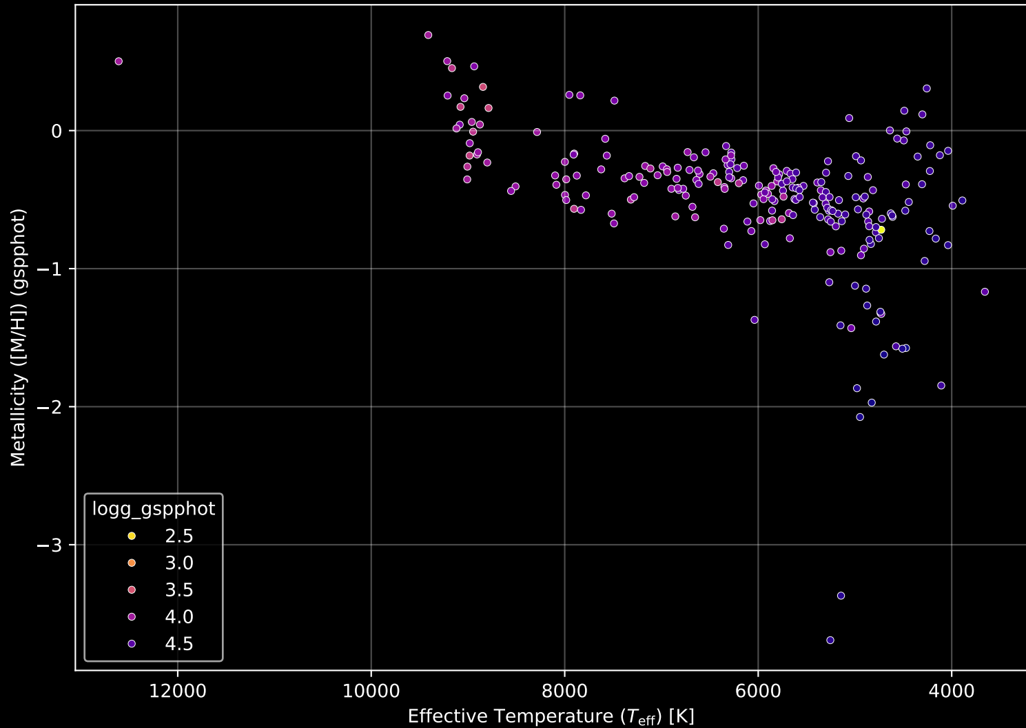
Gaia Cluster: [NGC_2428] Stellar Population Parameters (n= 234)
