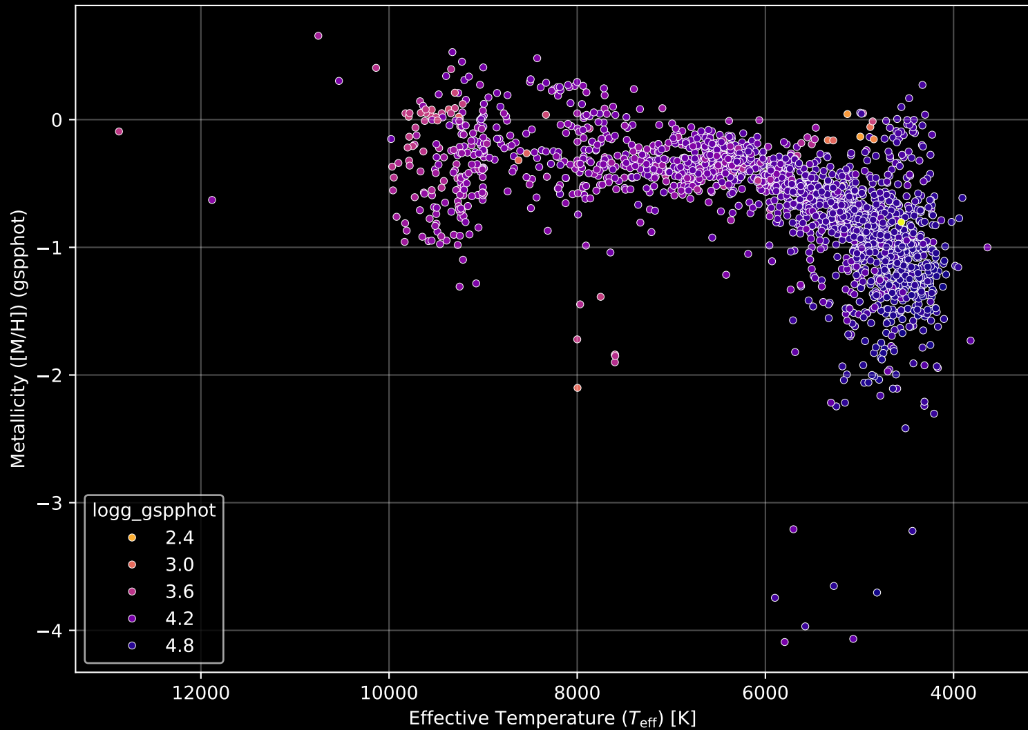
Gaia Cluster: [NGC_2437] Stellar Population Parameters (n= 1988)
