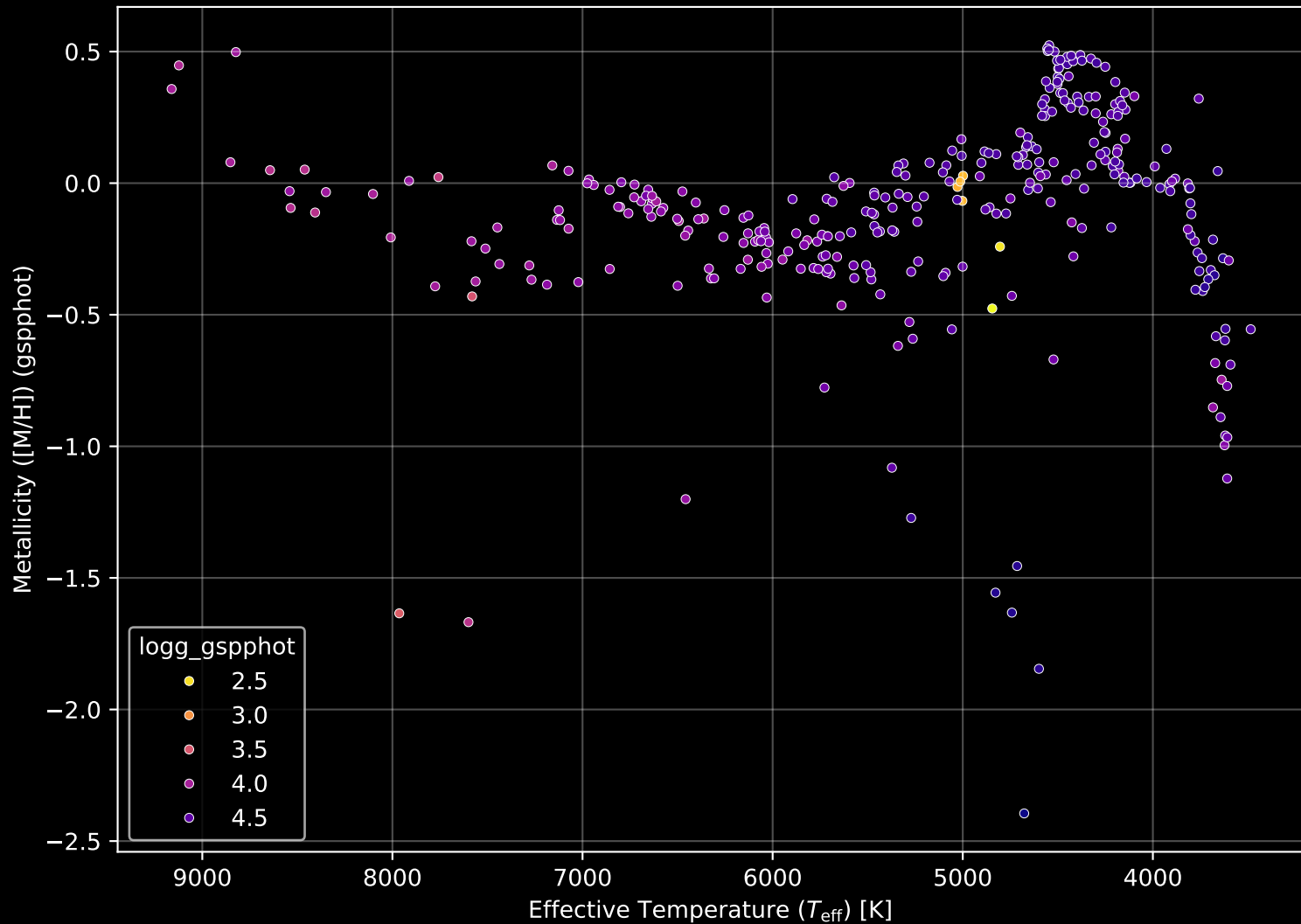
Gaia Cluster: [NGC_2527] Stellar Population Parameters (n= 330)
