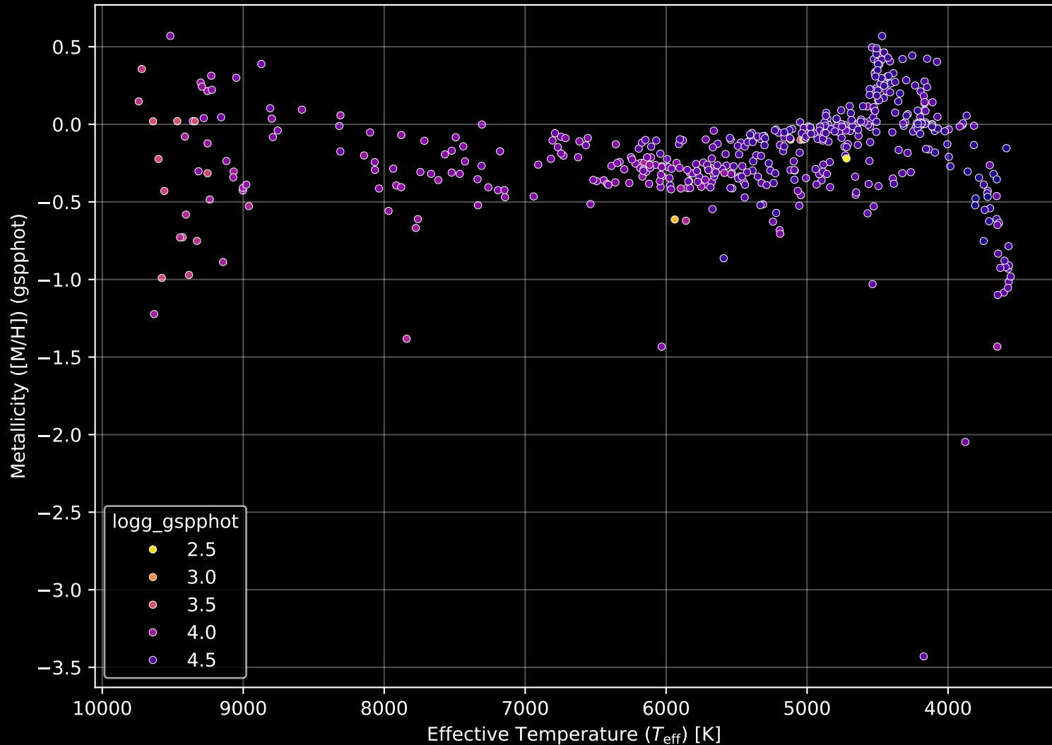
Gaia Cluster: [NGC_2548] Stellar Population Parameters (n= 490)
