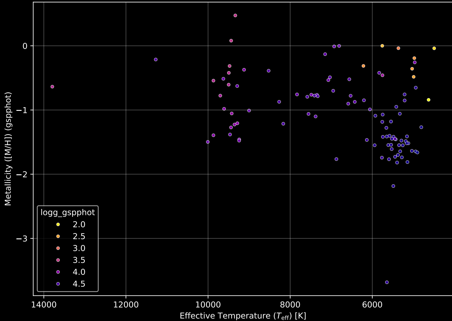
Gaia Cluster: [NGC_2580] Stellar Population Parameters (n= 101)
