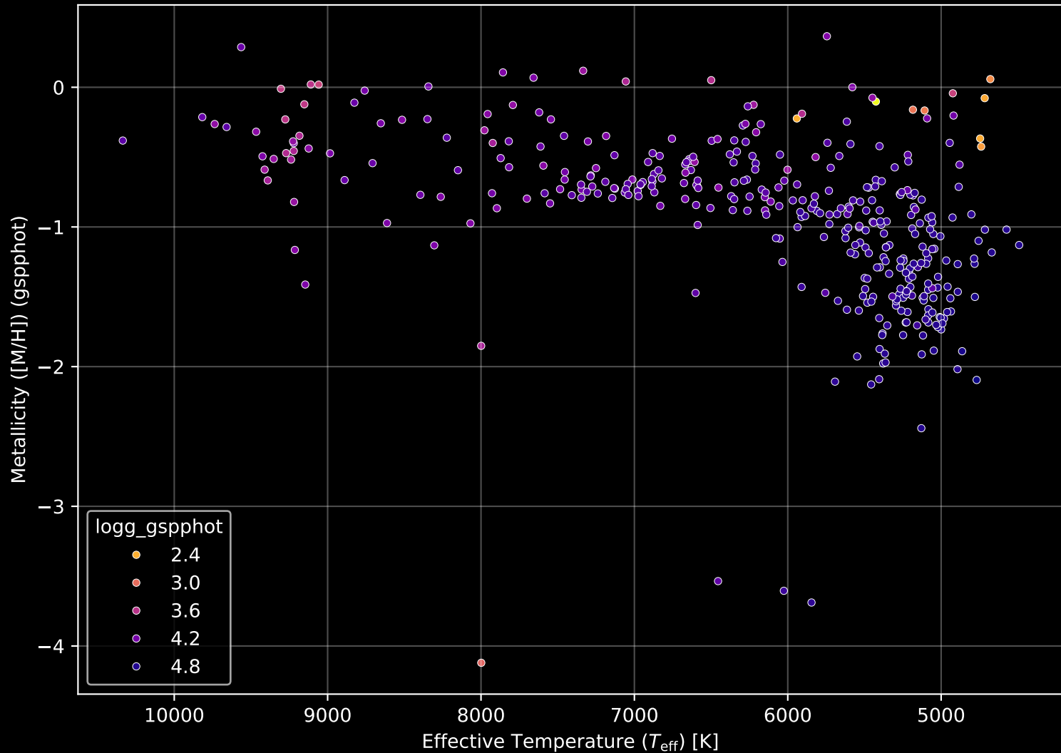
Gaia Cluster: [NGC_2587] Stellar Population Parameters (n= 377)
