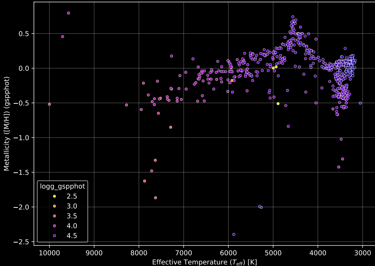
Gaia Cluster: [NGC_2632] Stellar Population Parameters (n= 545)
