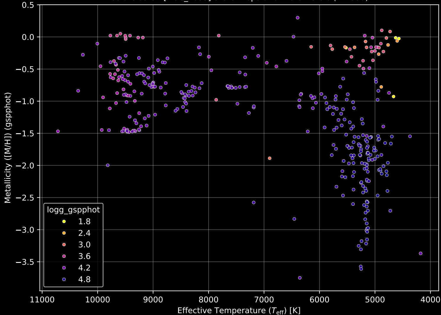
Gaia Cluster: [NGC_2635] Stellar Population Parameters (n= 359)
