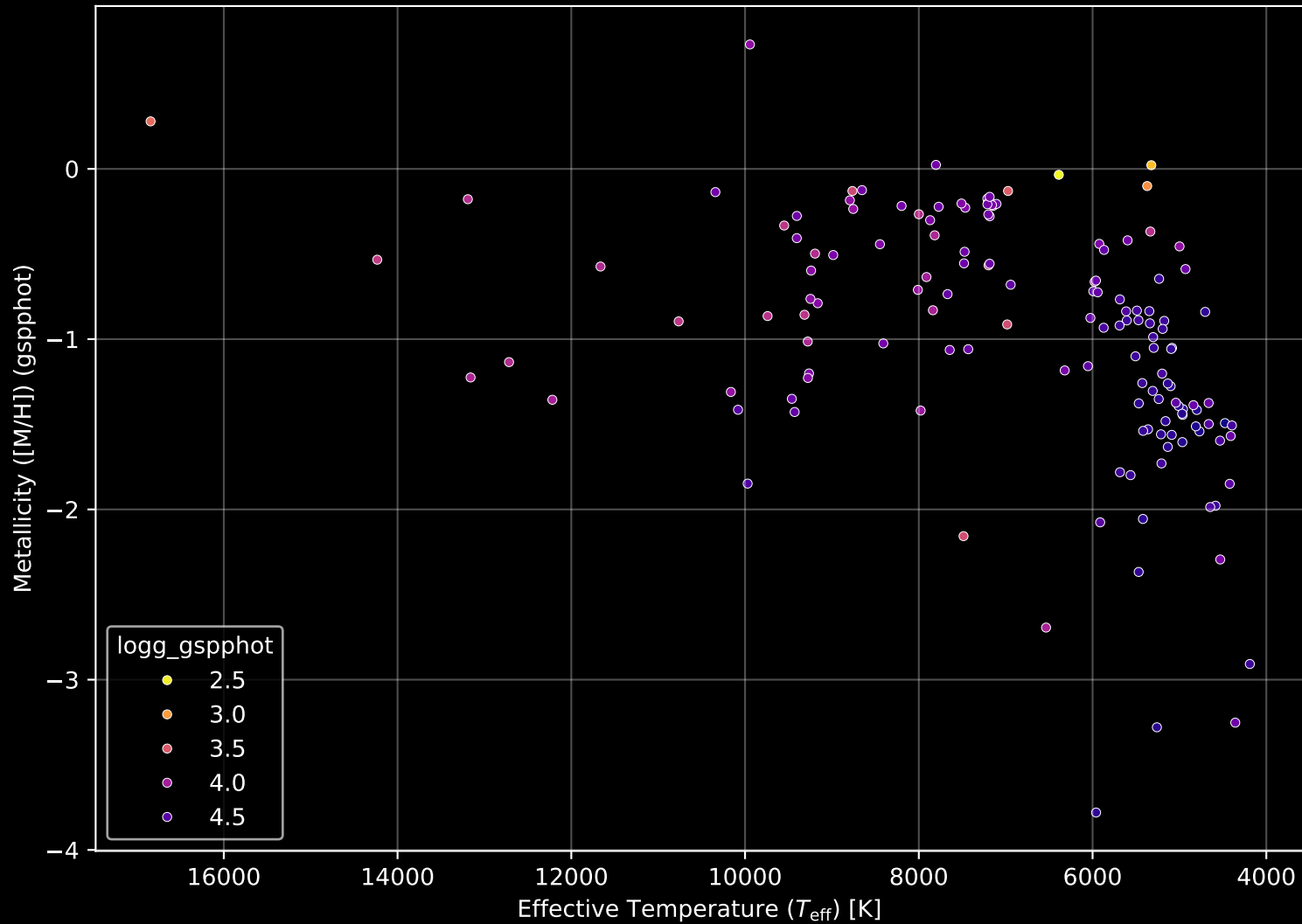
Gaia Cluster: [NGC_2659] Stellar Population Parameters (n= 145)
