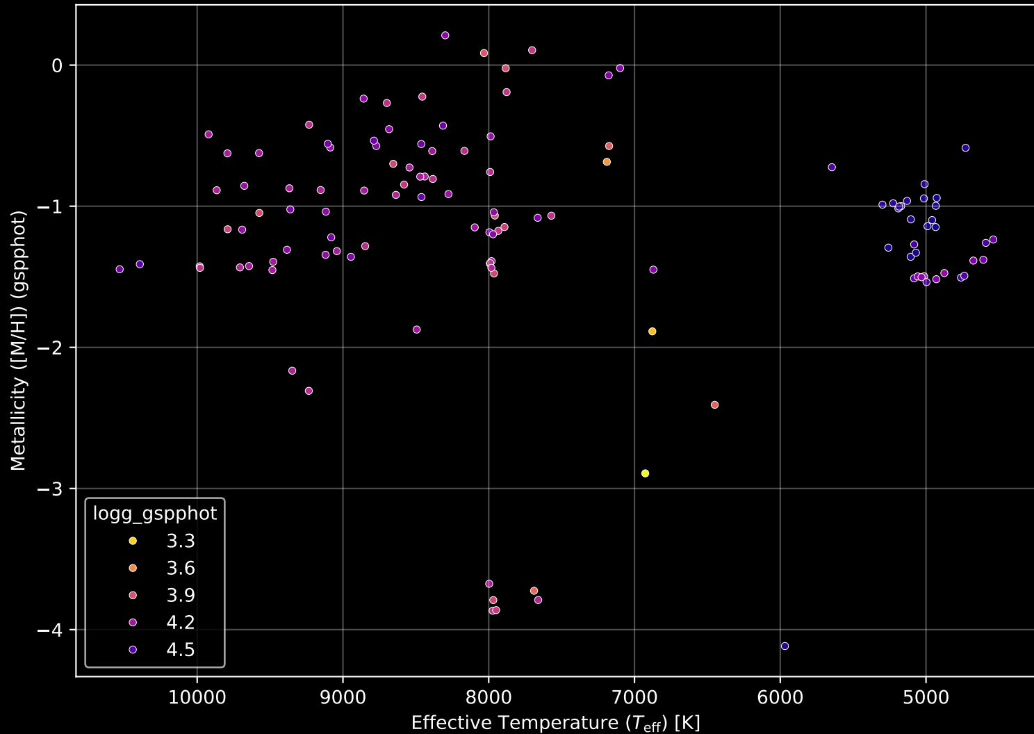
Gaia Cluster: [NGC_2671] Stellar Population Parameters (n= 121)
