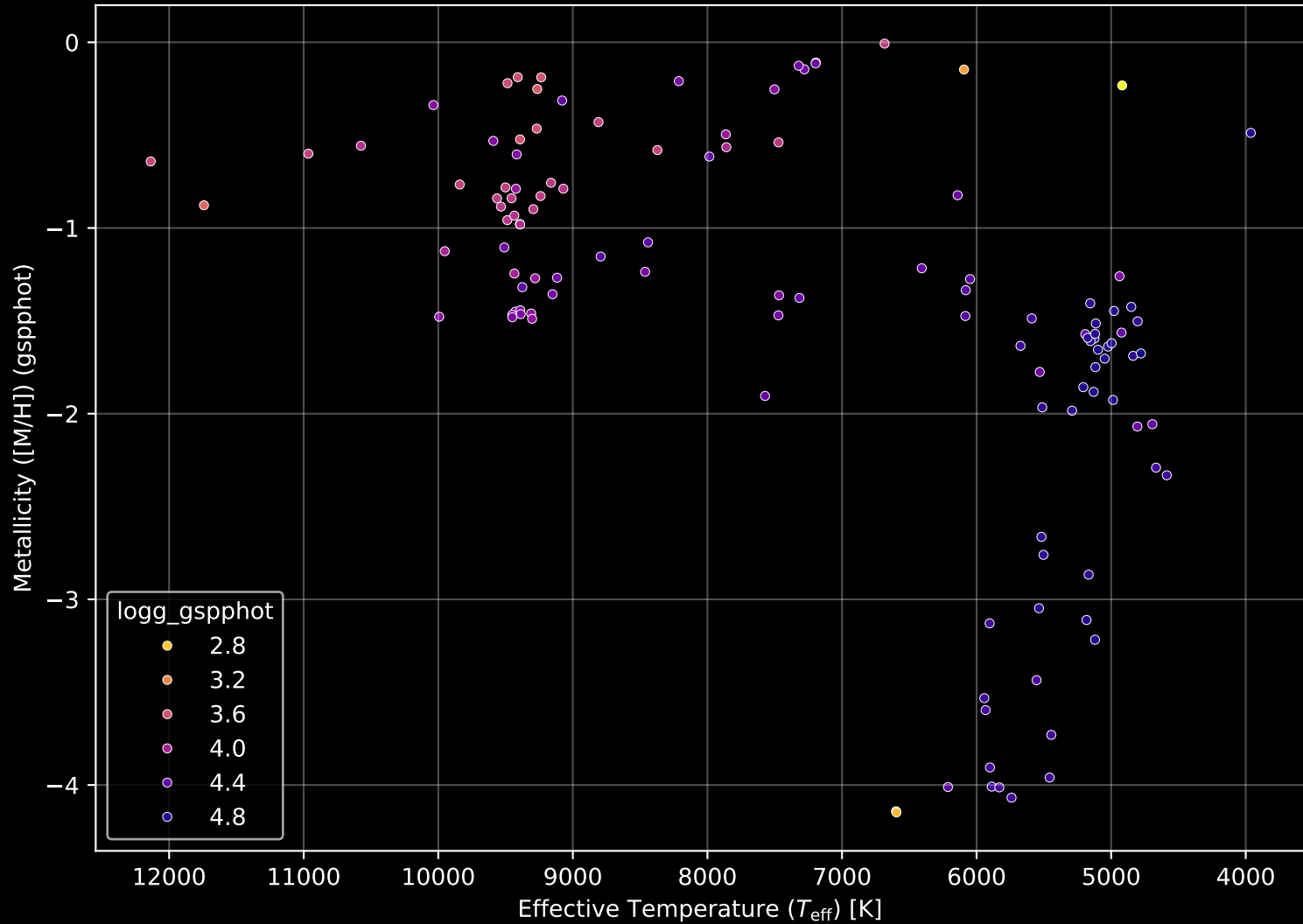
Gaia Cluster: [NGC_2866] Stellar Population Parameters (n= 121)
