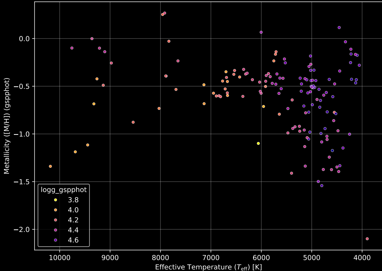
Gaia Cluster: [NGC_2910] Stellar Population Parameters (n= 147)
