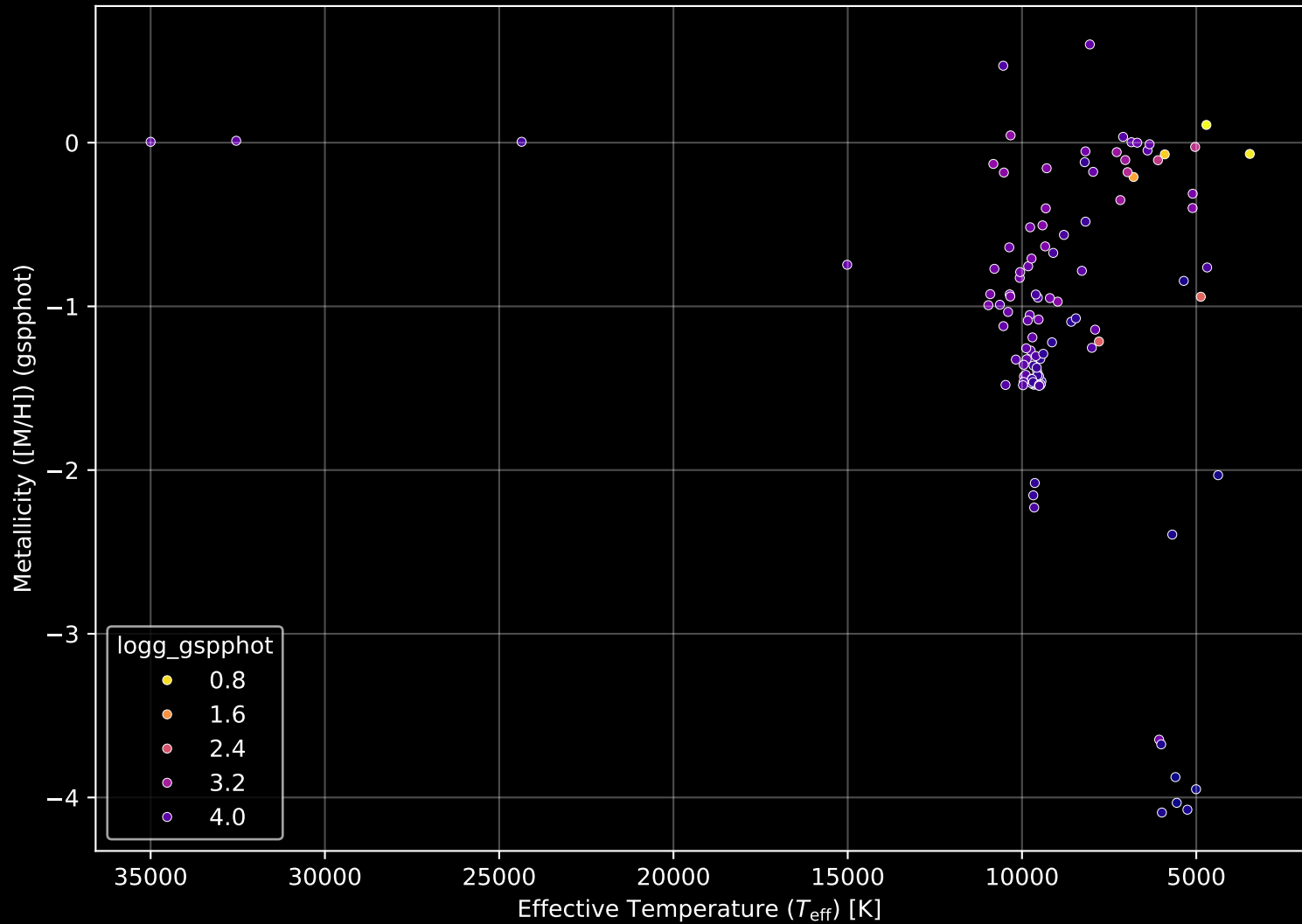
Gaia Cluster: [NGC_3105] Stellar Population Parameters (n= 116)
