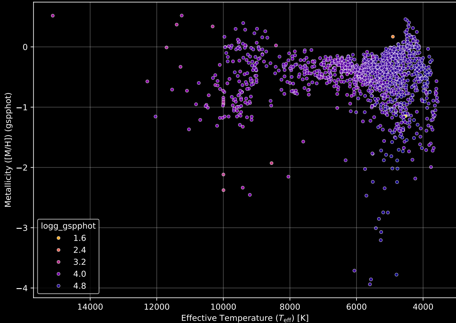
Gaia Cluster: [NGC_3114] Stellar Population Parameters (n= 1432)
