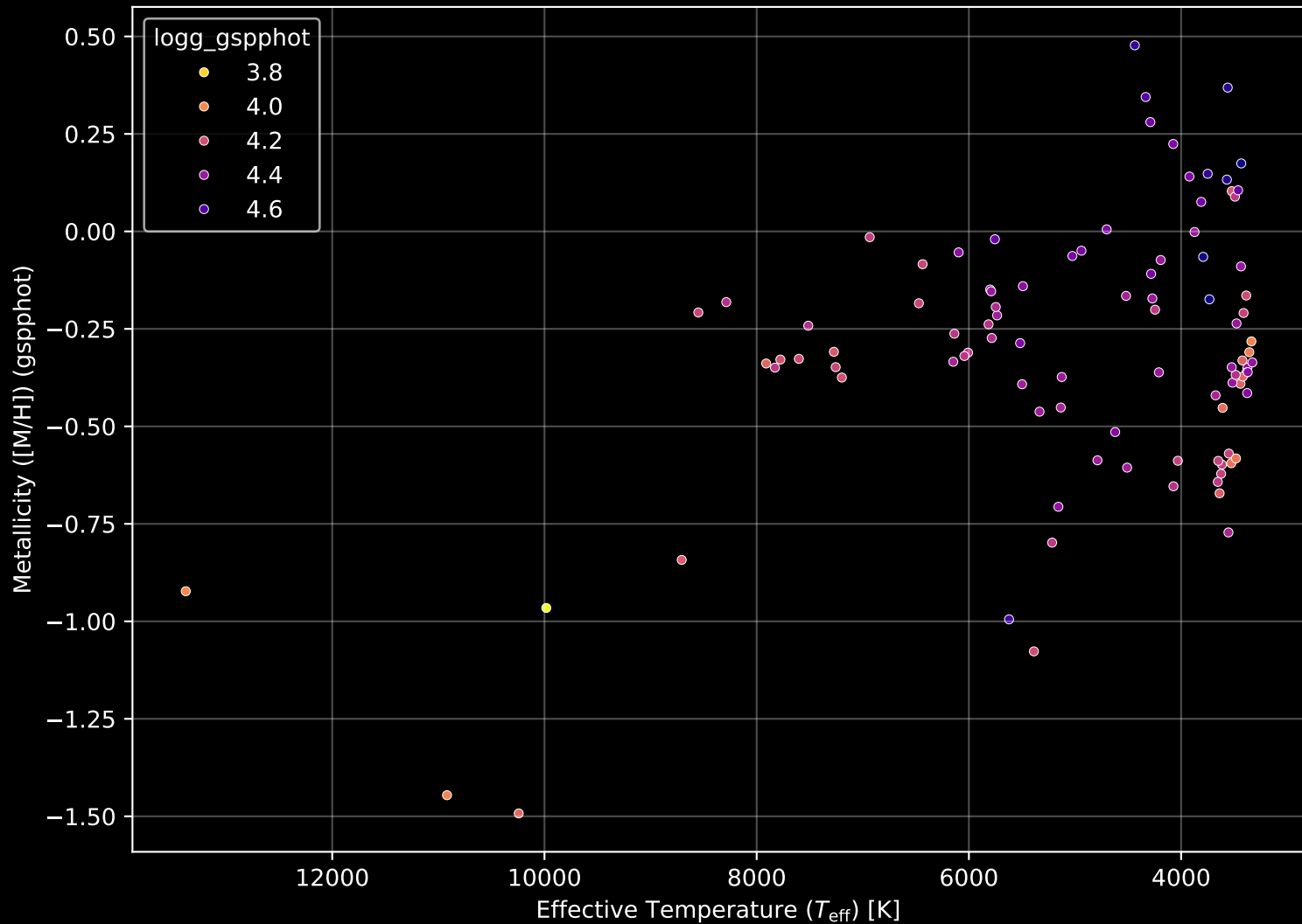
Gaia Cluster: [NGC_3228] Stellar Population Parameters (n= 98)
