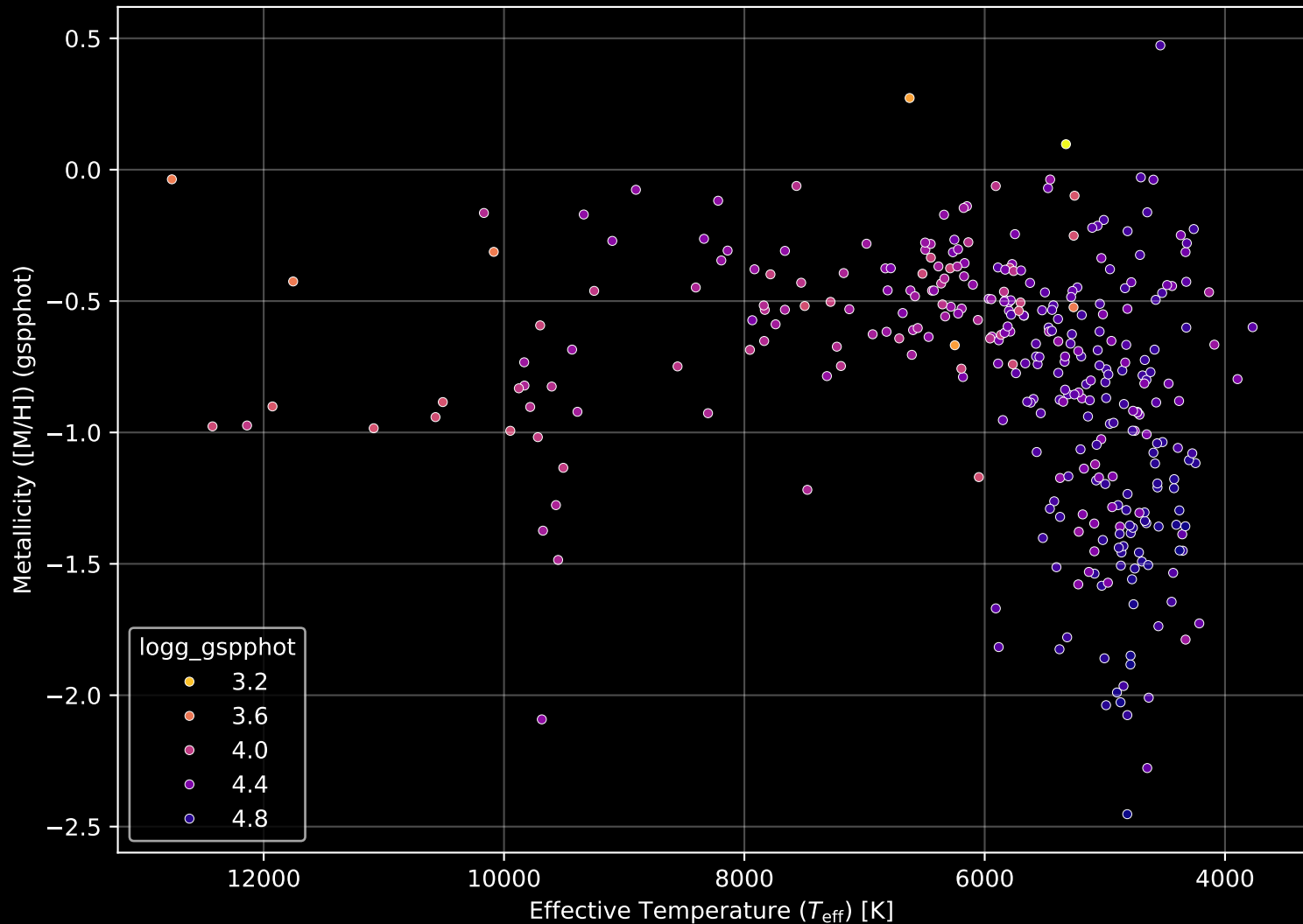
Gaia Cluster: [NGC_3330] Stellar Population Parameters (n= 331)
