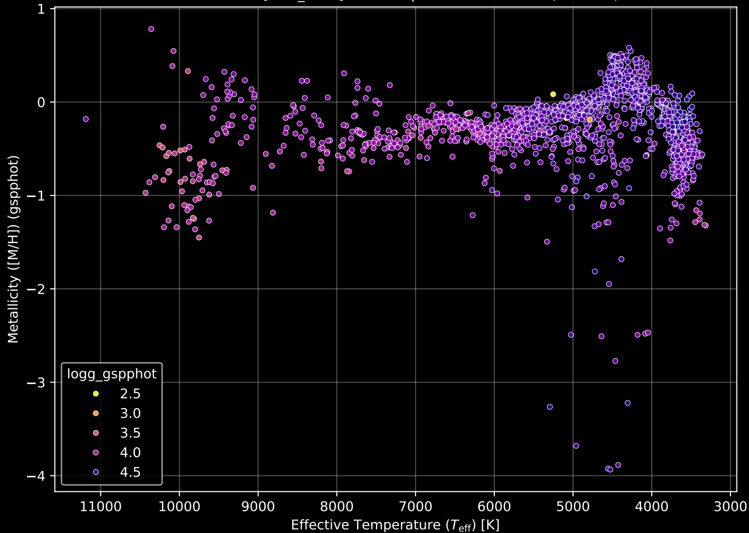
Gaia Cluster: [NGC_3532] Stellar Population Parameters (n= 1694)
