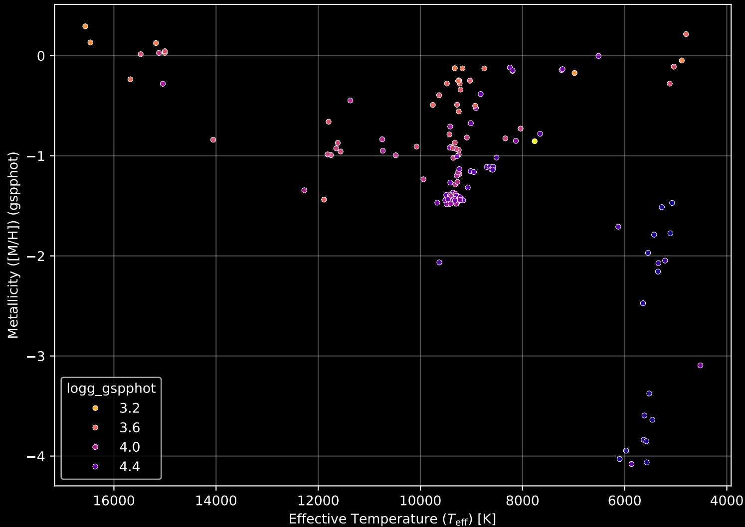
Gaia Cluster: [NGC_366] Stellar Population Parameters (n= 140)
