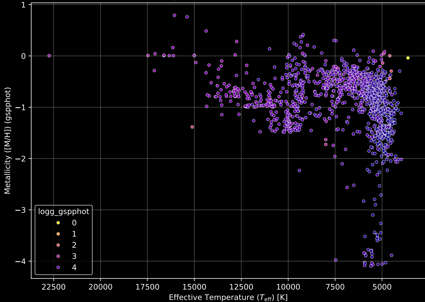
Gaia Cluster: [NGC_3766] Stellar Population Parameters (n= 1197)
