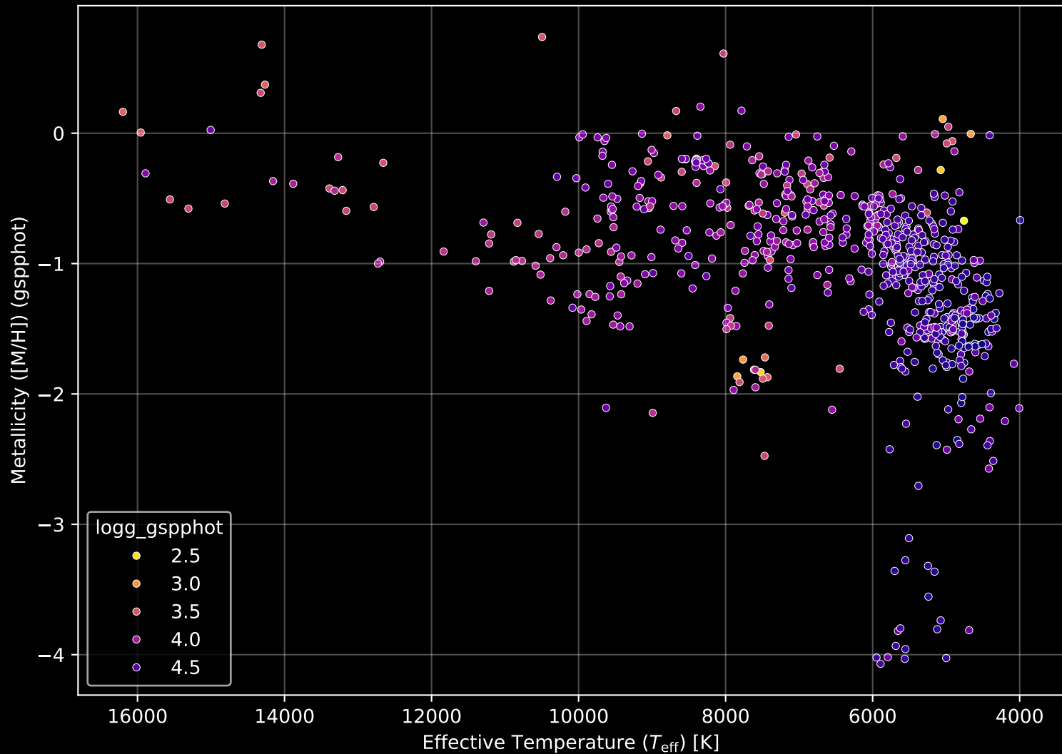
Gaia Cluster: [NGC_4103] Stellar Population Parameters (n= 729)
