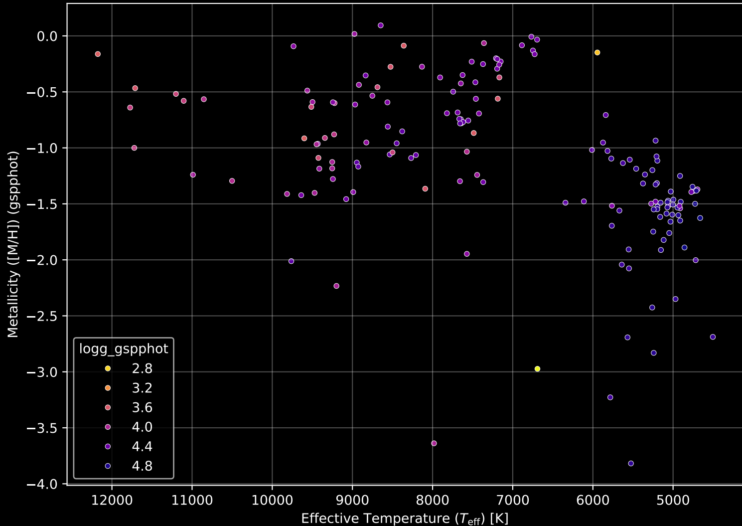
Gaia Cluster: [NGC_433] Stellar Population Parameters (n= 162)
