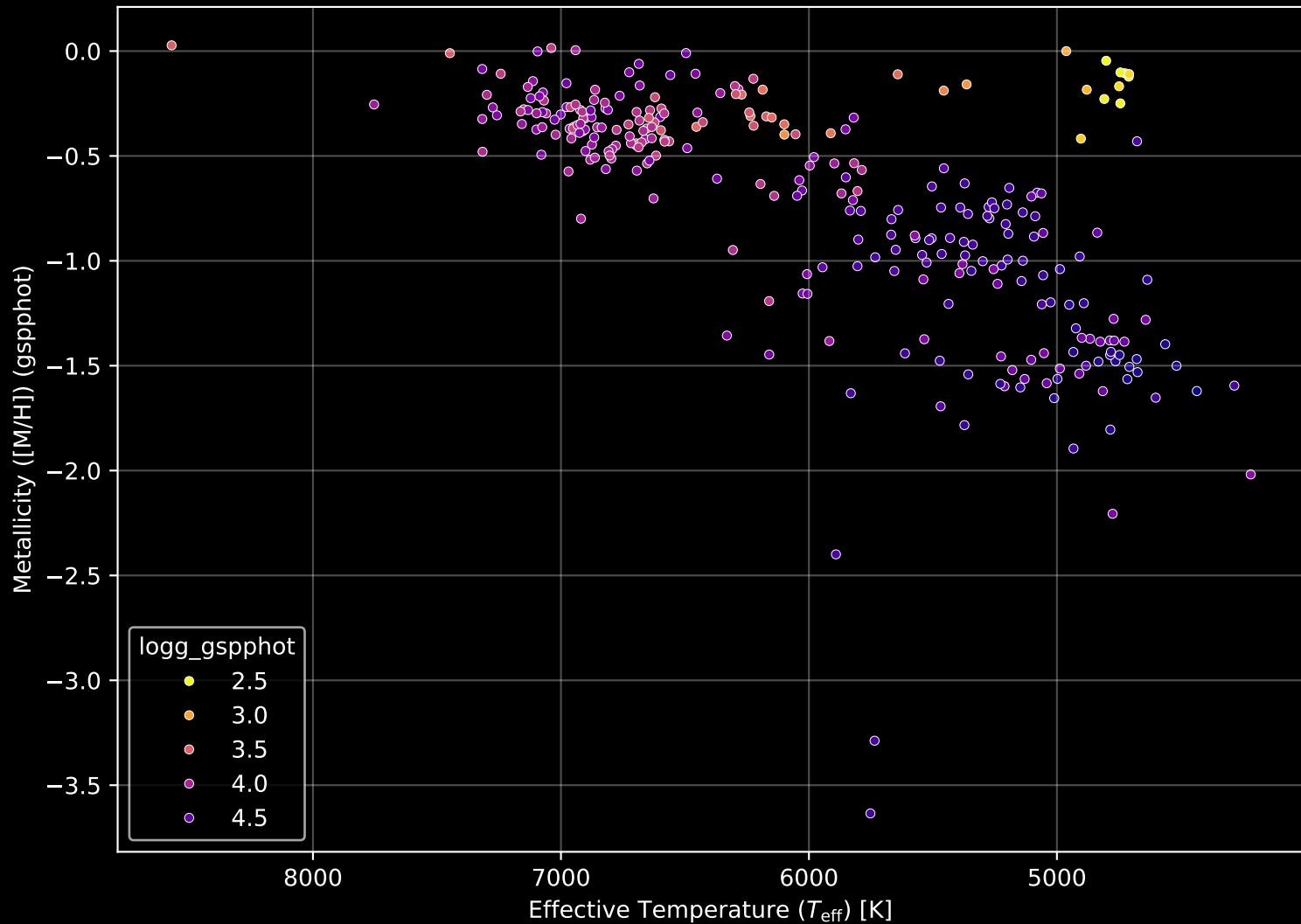
Gaia Cluster: [NGC_4337] Stellar Population Parameters (n= 287)
