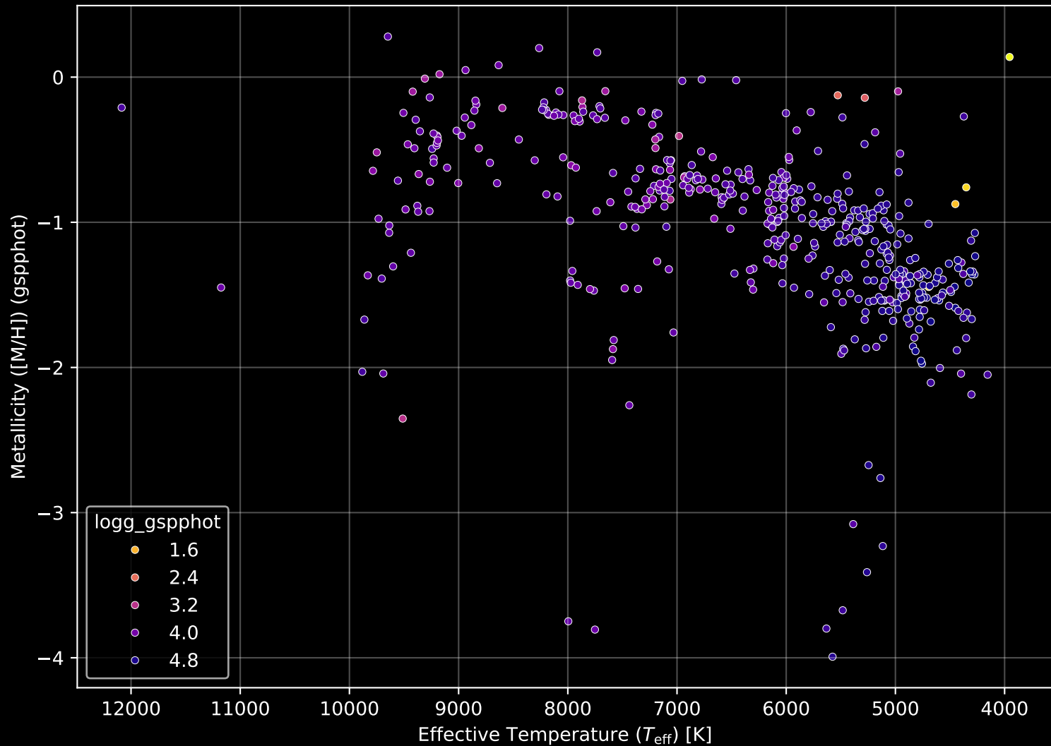
Gaia Cluster: [NGC_4349] Stellar Population Parameters (n= 482)
