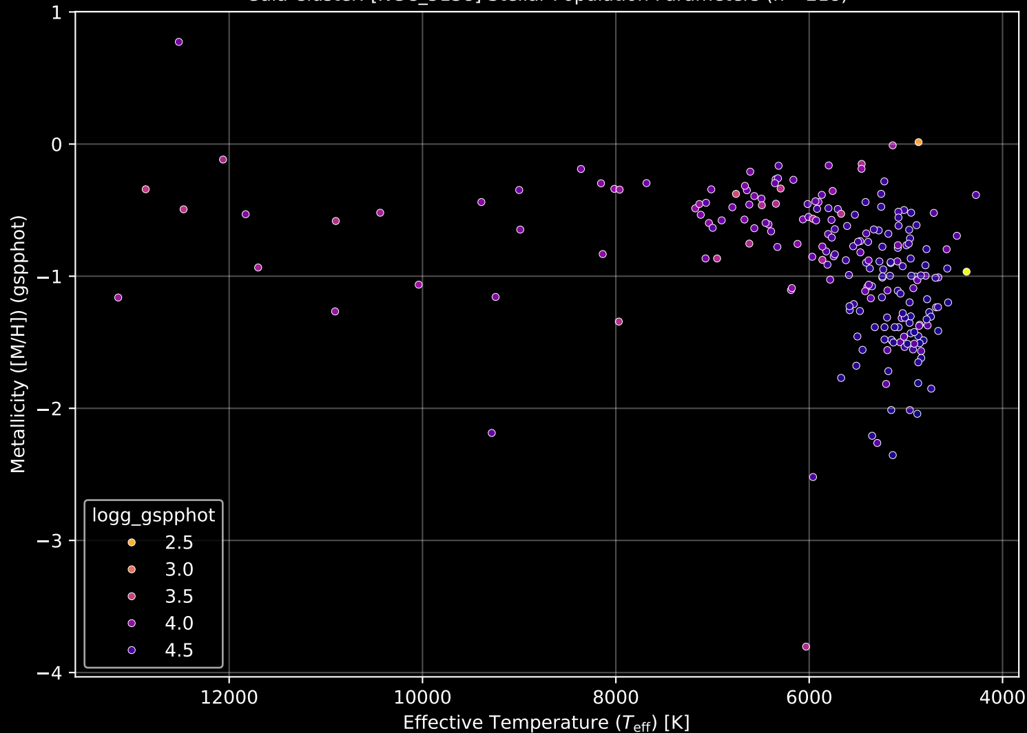
Gaia Cluster: [NGC_5138] Stellar Population Parameters (n= 218)
