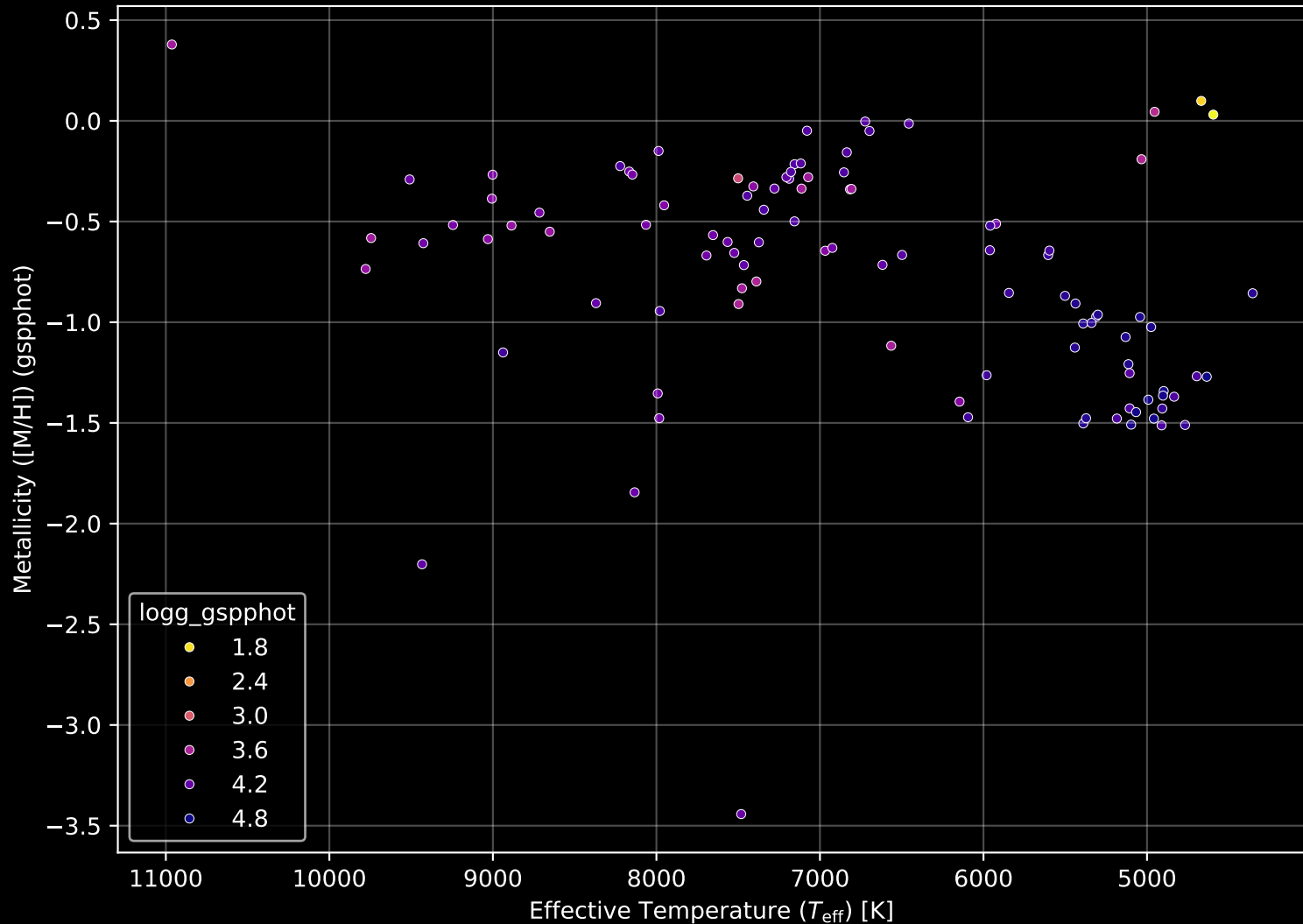
Gaia Cluster: [NGC_5269] Stellar Population Parameters (n= 103)
