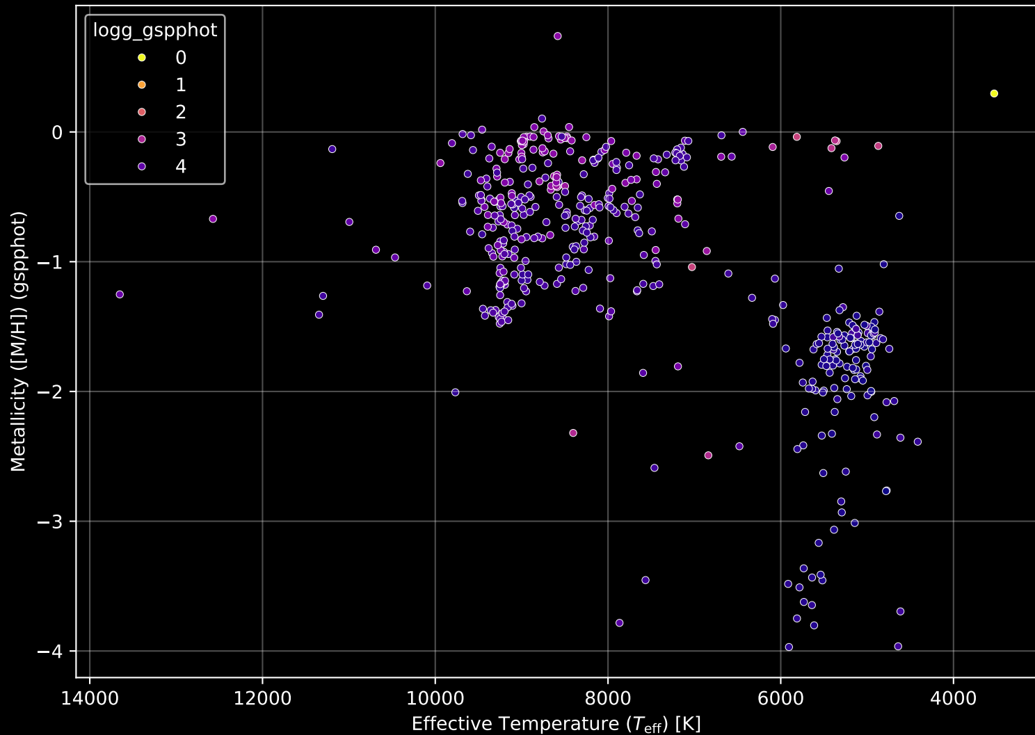
Gaia Cluster: [NGC_559] Stellar Population Parameters (n= 492)
