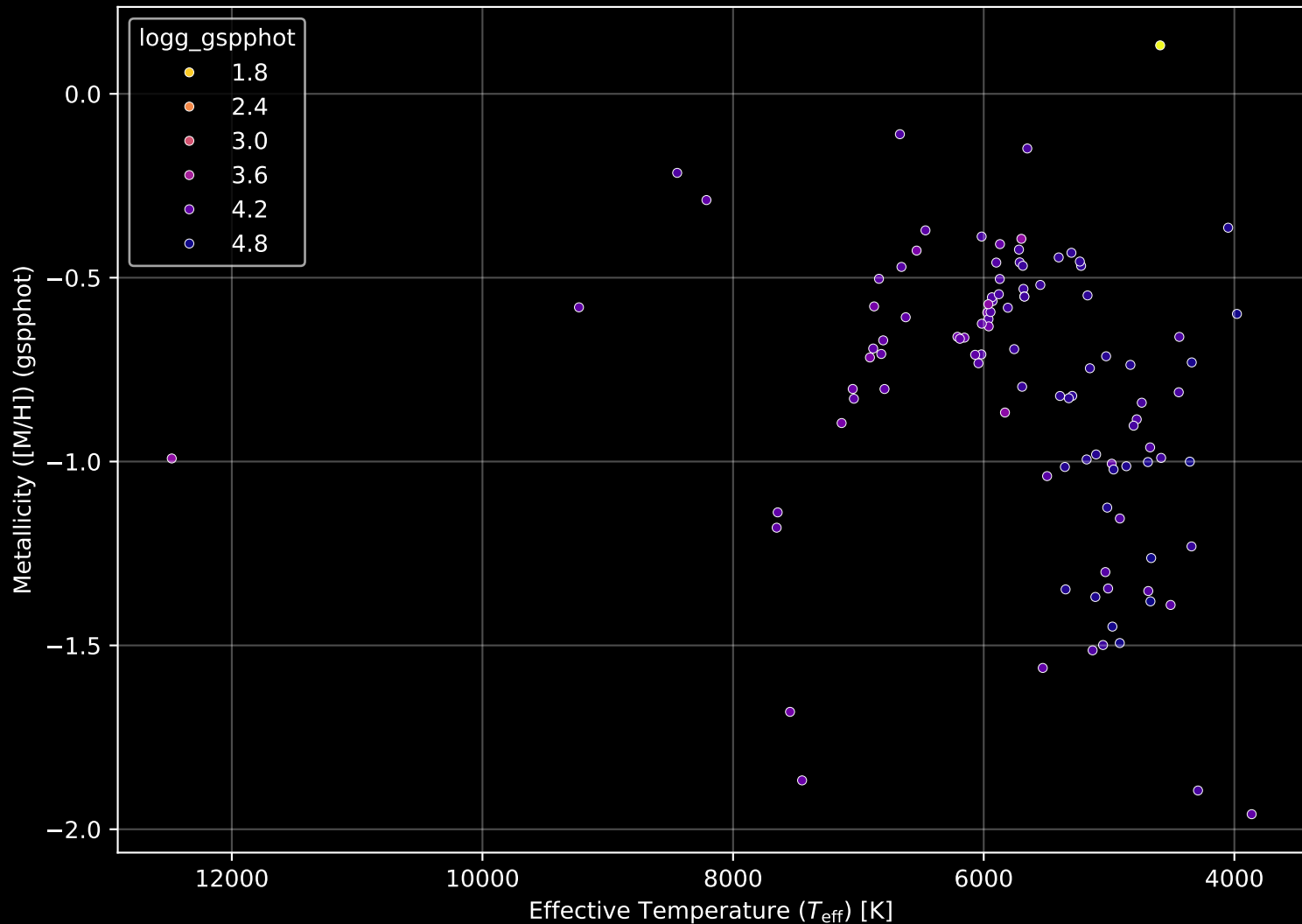
Gaia Cluster: [NGC_5749] Stellar Population Parameters (n= 104)
