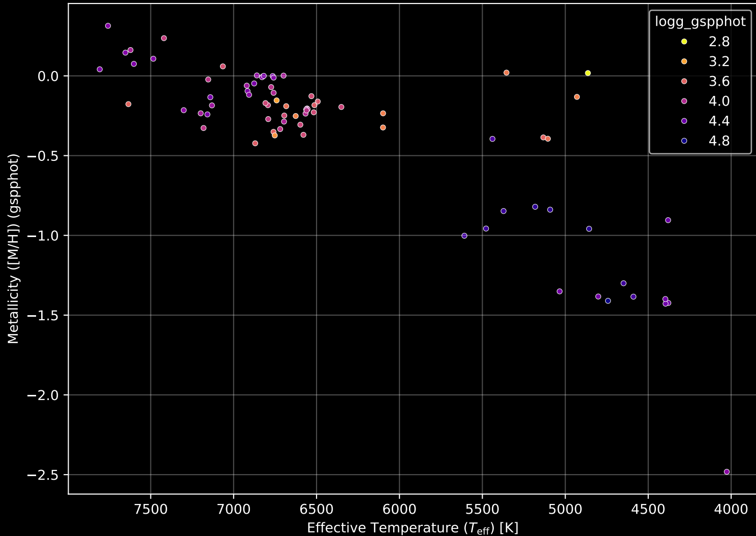
Gaia Cluster: [NGC_5764] Stellar Population Parameters (n= 77)
