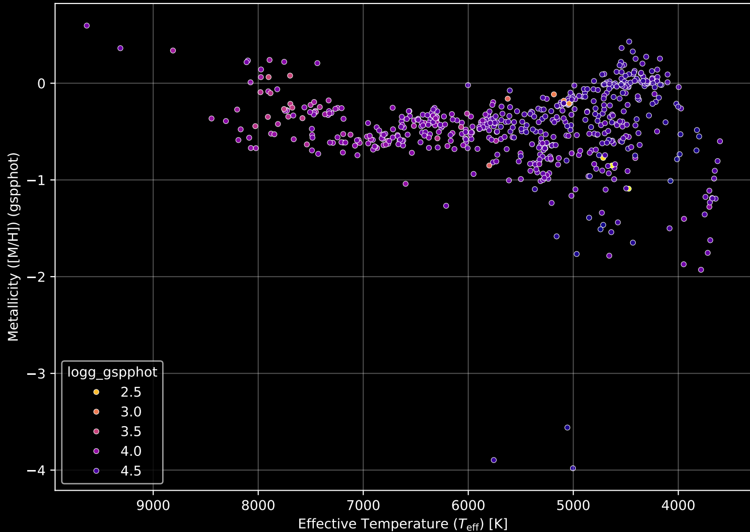
Gaia Cluster: [NGC_5822] Stellar Population Parameters (n= 609)
