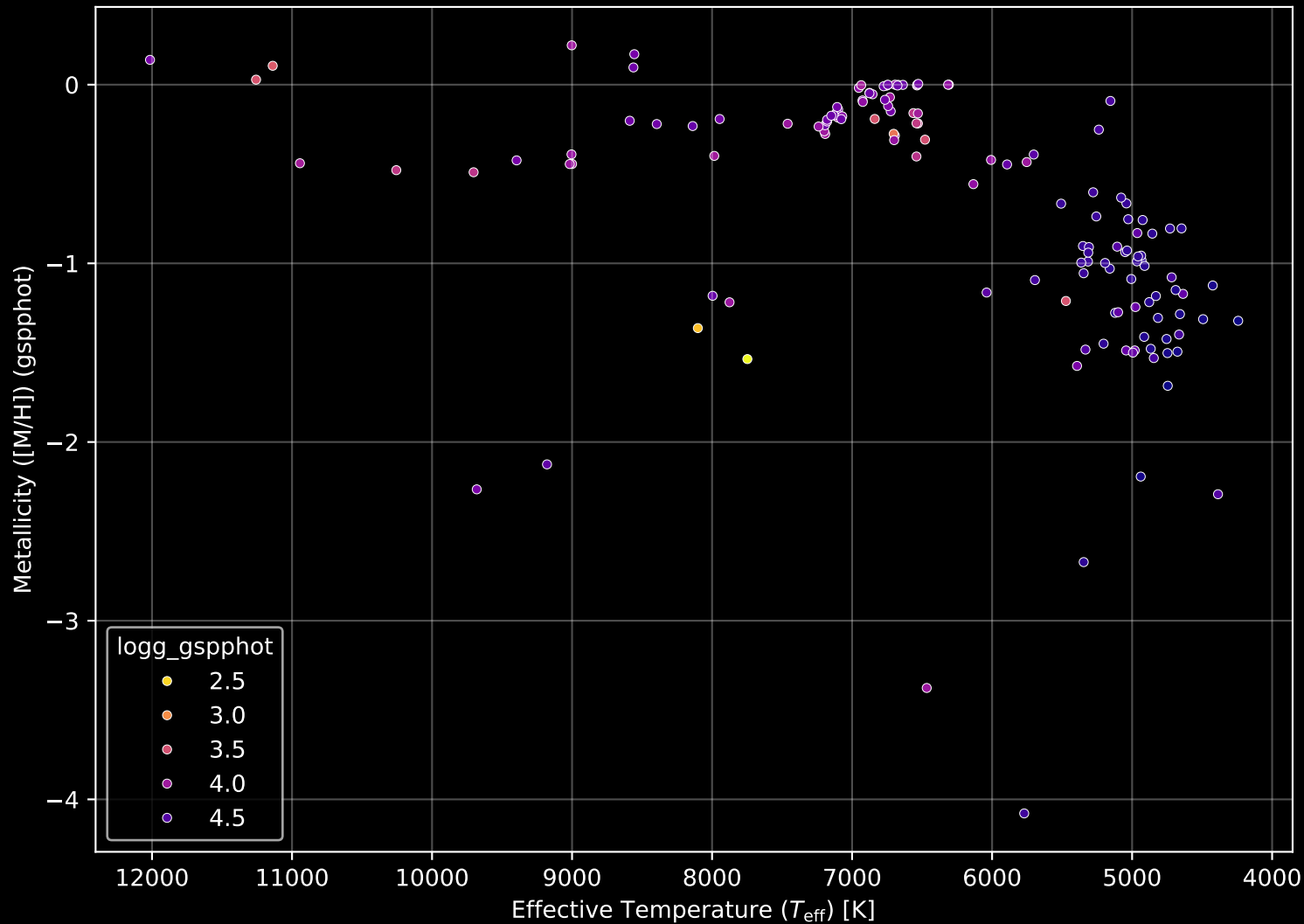
Gaia Cluster: [NGC_6031] Stellar Population Parameters (n= 144)
