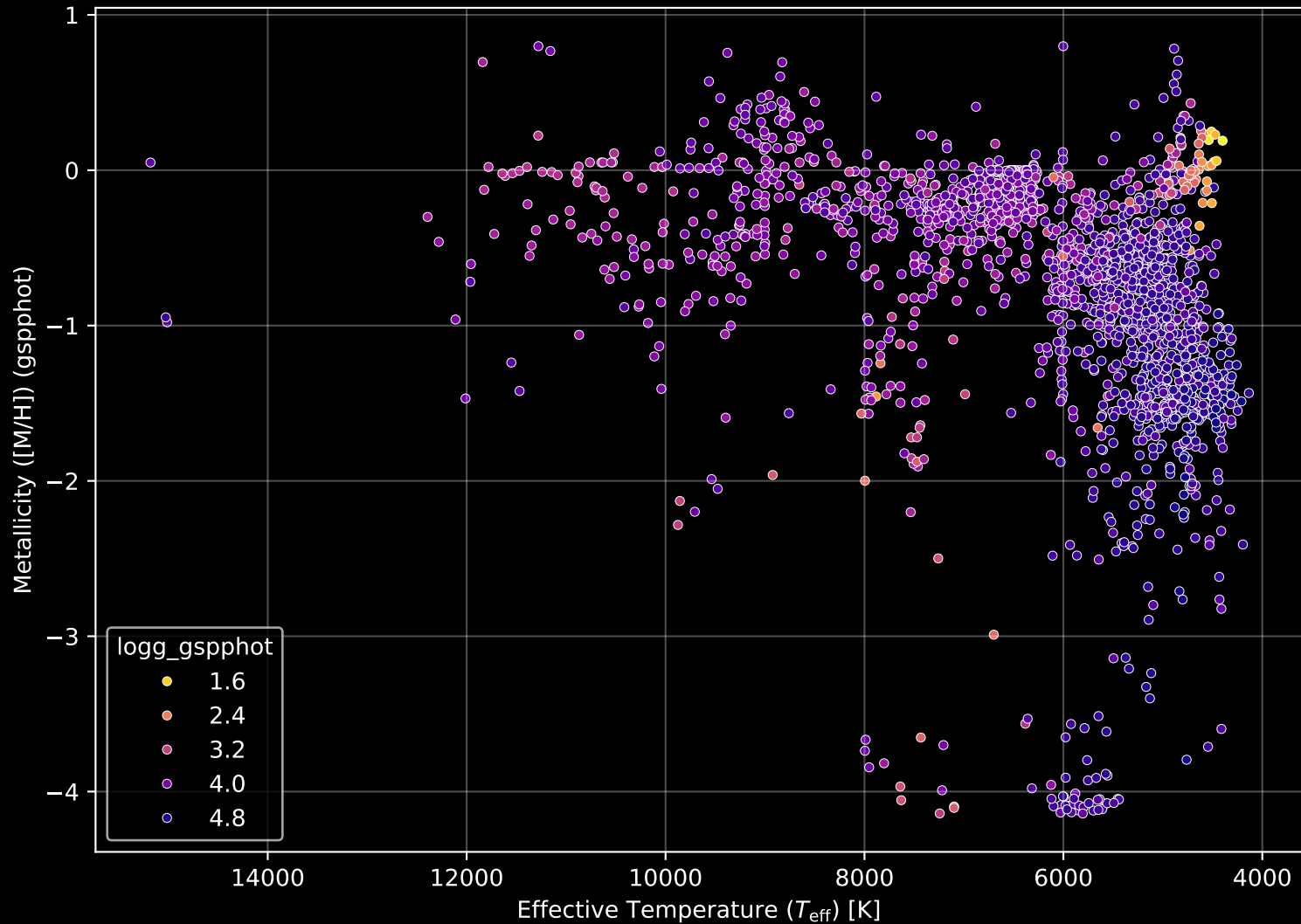
Gaia Cluster: [NGC_6067] Stellar Population Parameters (n= 2021)
