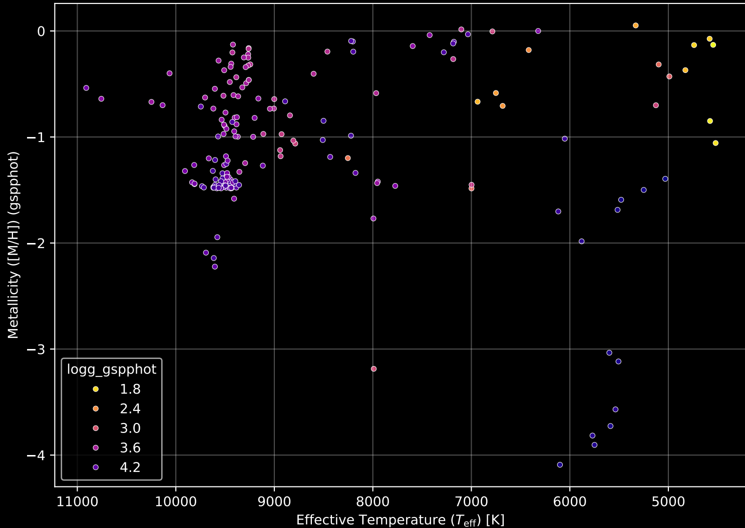
Gaia Cluster: [NGC_609] Stellar Population Parameters (n= 192)
