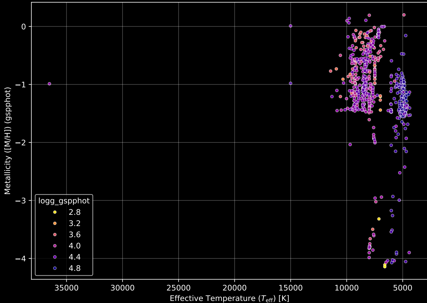
Gaia Cluster: [NGC_6167] Stellar Population Parameters (n= 621)
