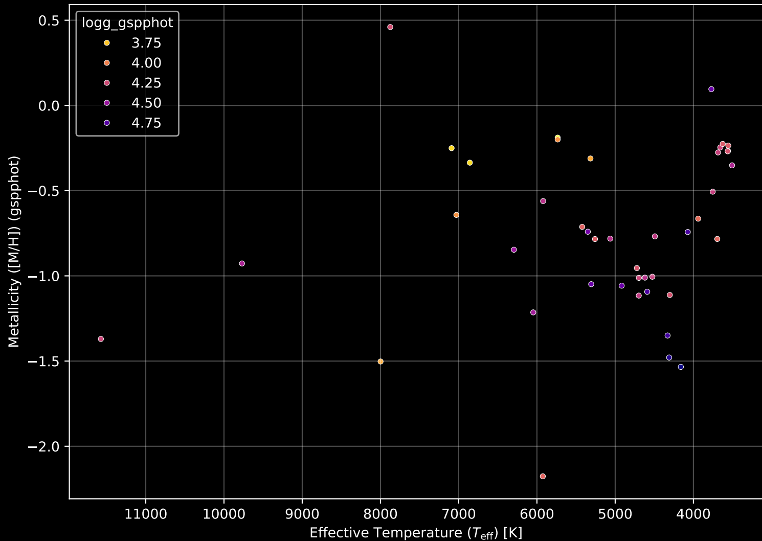
Gaia Cluster: [NGC 6178] Stellar Population Parameters (n= 43)
